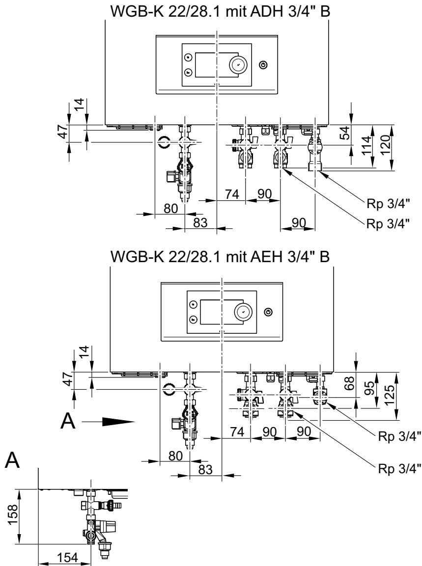
Abb. 12: WGB-K 22/28.1 mit ADH/AEH
