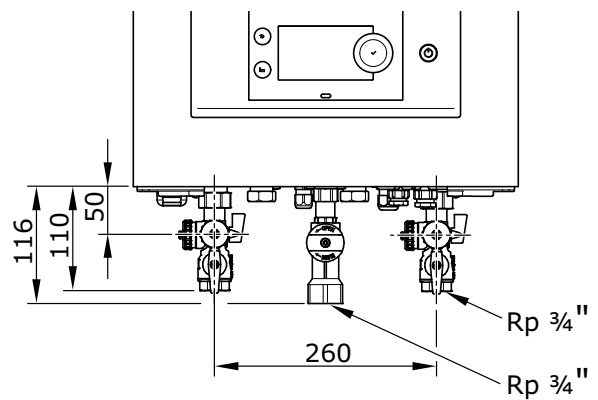
WGB 38.1 mit ADH 2 B
