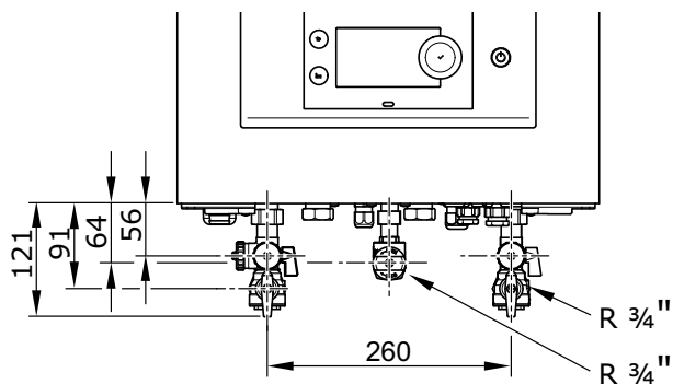
WGB 14.1/22.1/28.1 mit AEH ¾" B
