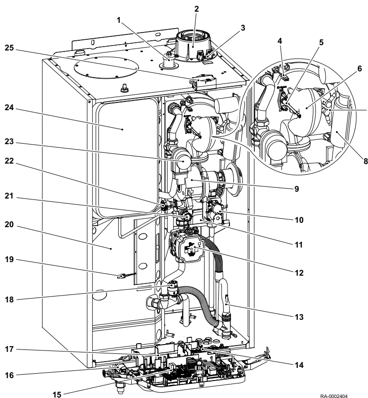
Abb. 2: WGB-K 22/28.1 (dargestellt ohne Vorderwand und Abdeckung der Regelung)
