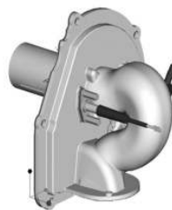
Abb. 4: Vormischkanal – Gas-Brennwertgeräte mit EVolution-Technik
