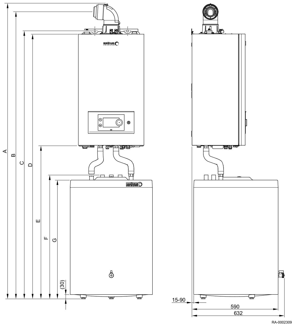
Abb. 10: WGB 14.1–38.1 mit BS-Speicher
