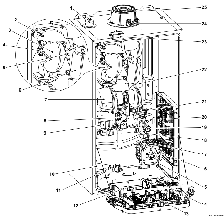
Abb. 1: WGB 14.1–38.1 (dargestellt ohne Vorderwand und Abdeckung der Regelung)
