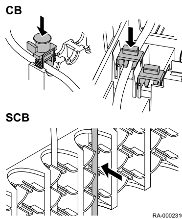
Abb. 18: Zugentlastungen Anschlussleiterplatte CB/Erweiterungsleiterplatte SCB
