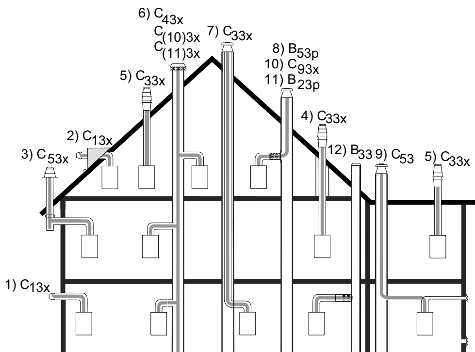
Abb. 29: Anschlussmöglichkeiten mit KAS (Zubehör)
