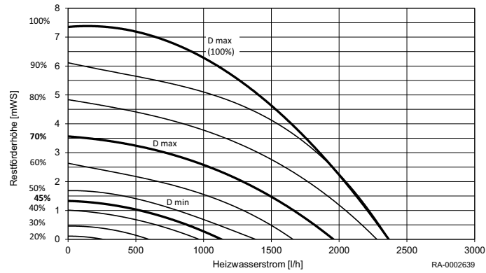
Abb. 14: Restförderhöhe WGB 14.1–22.1
