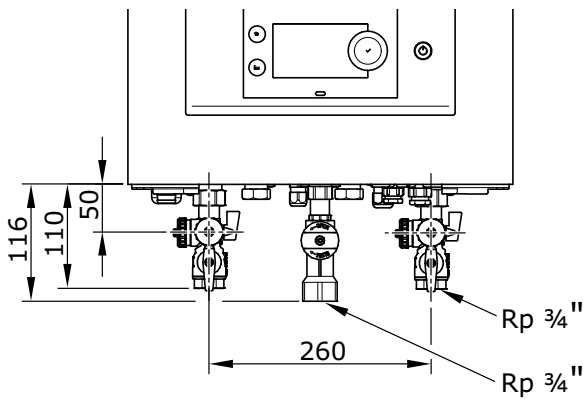
WGB 14.1/22.1/28.1 mit ADH ¾" B
