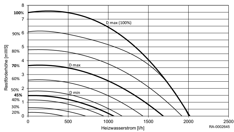
Abb. 17: Restförderhöhe WGB-K 22/28.1
